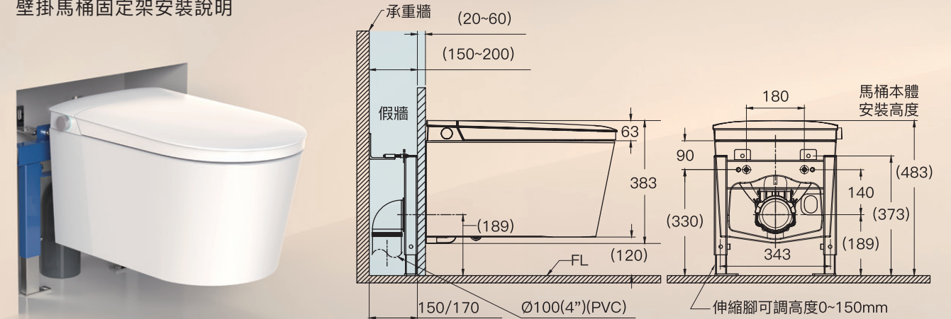
壁掛馬桶固定架安裝說明
